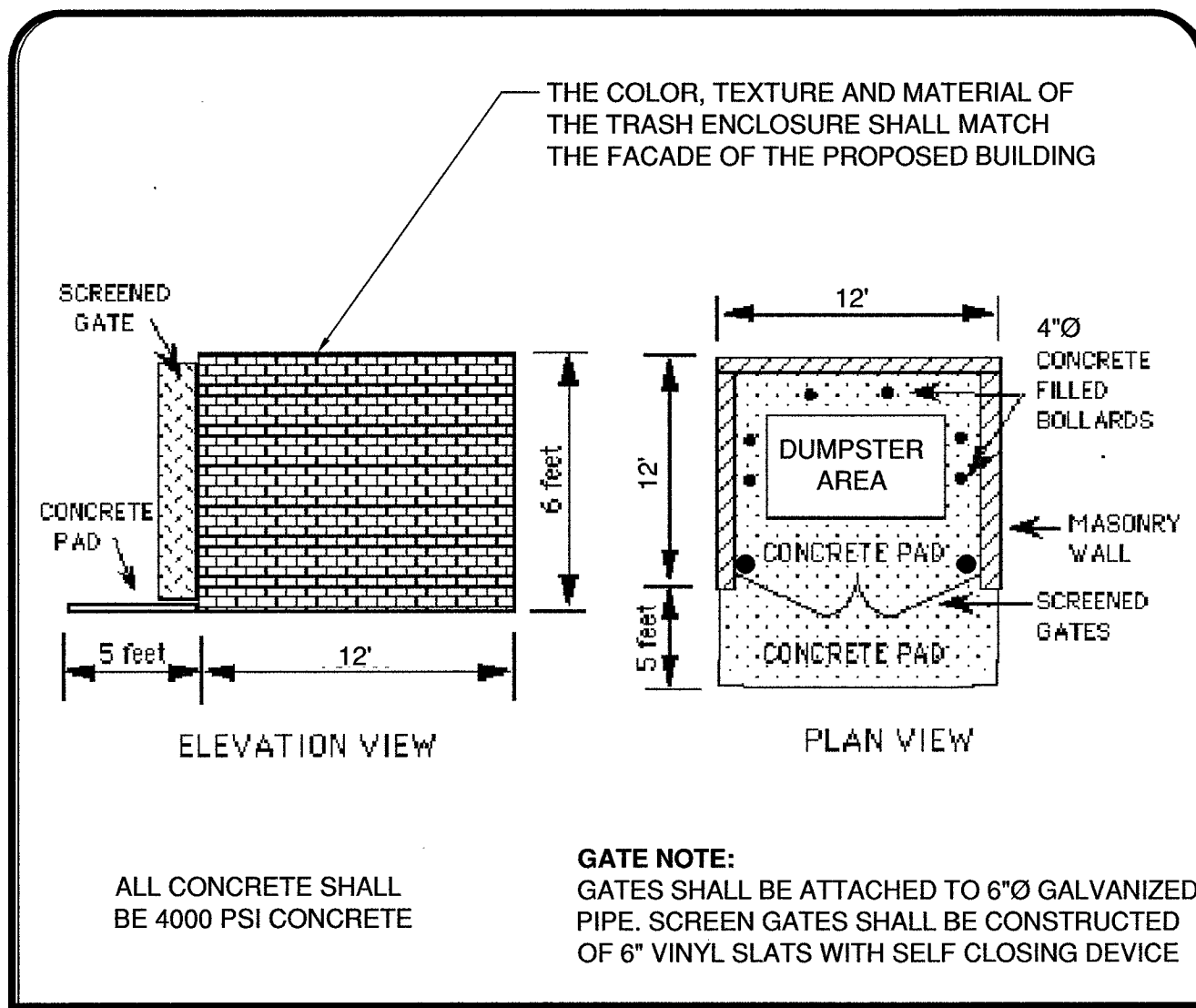
MASONRY TRASH ENCLOSURE DETAIL N.T.S.
