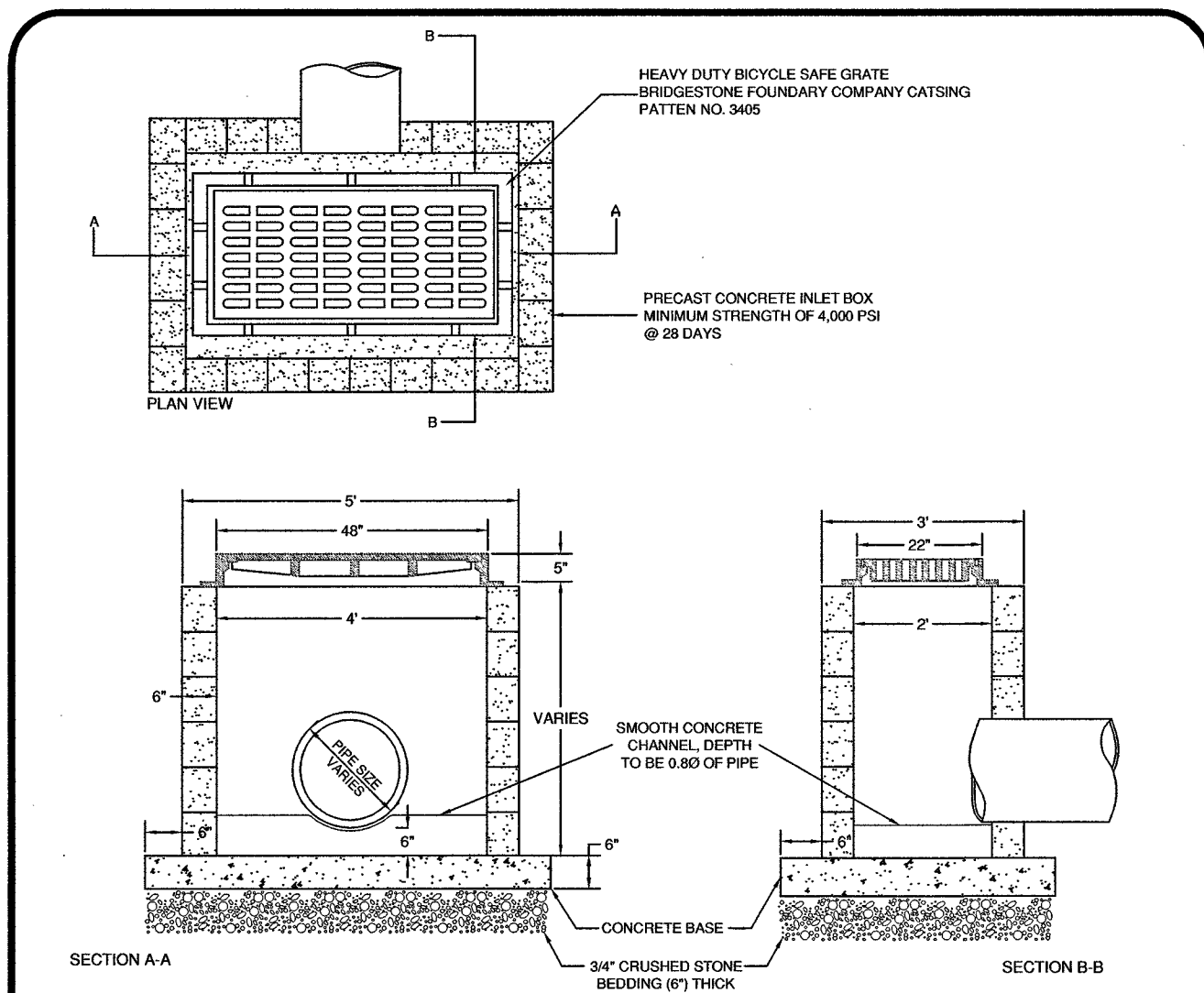
TYPE A INLET DETAIL N.T.S.
