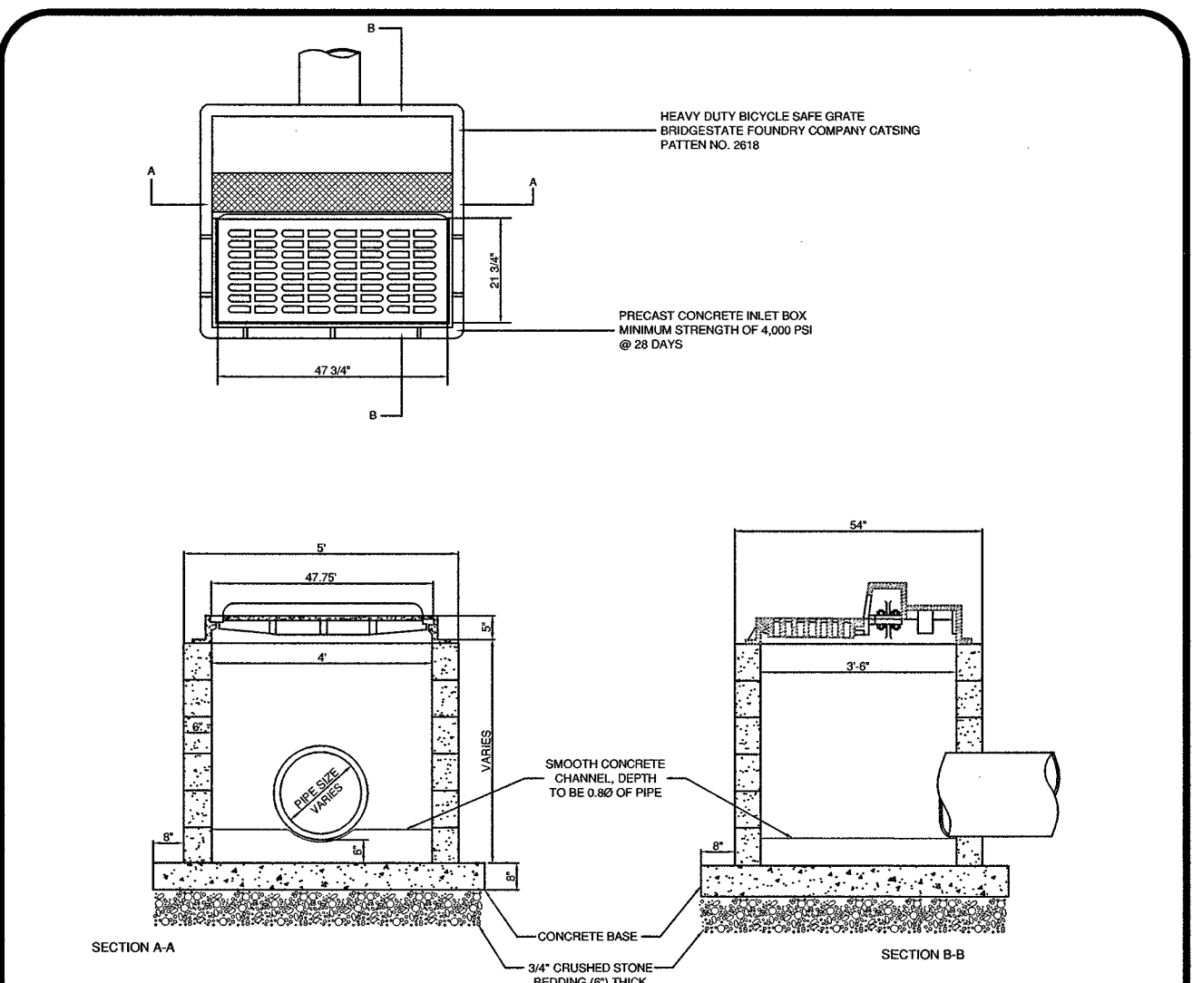
TYPE B INLET DETAIL N.T.S.
