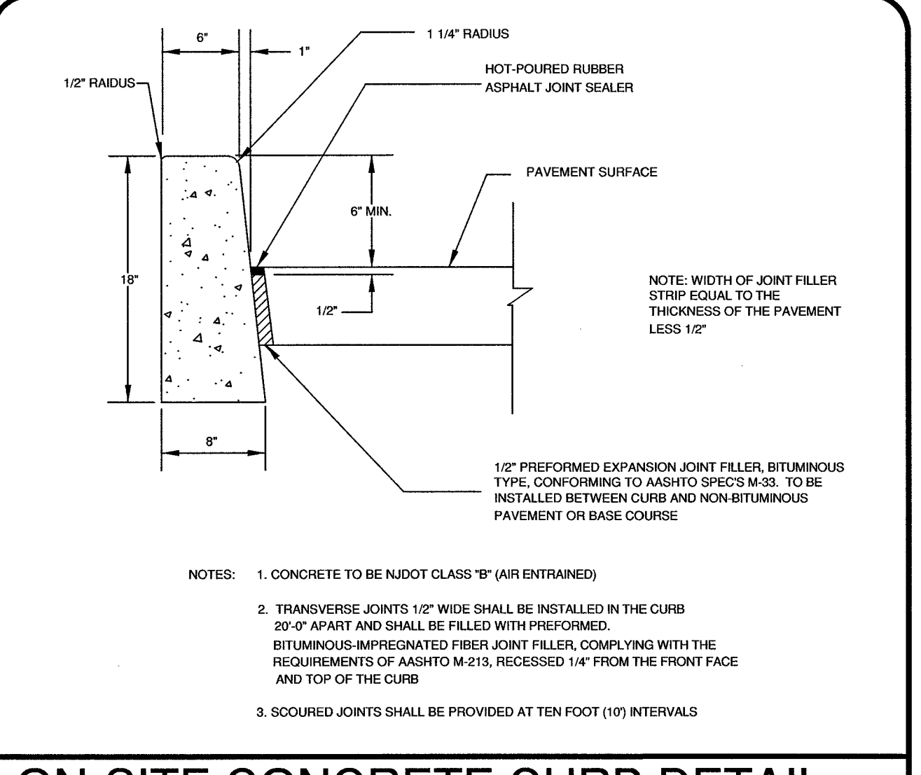
ON-SITE CONCRETE CURB DETAIL N.T.S.
