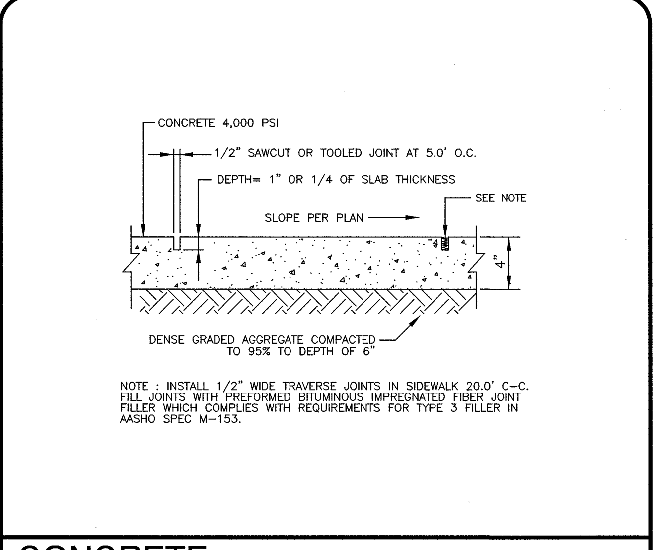
CONCRETE SIDEWALK DETAIL N.T.S.
